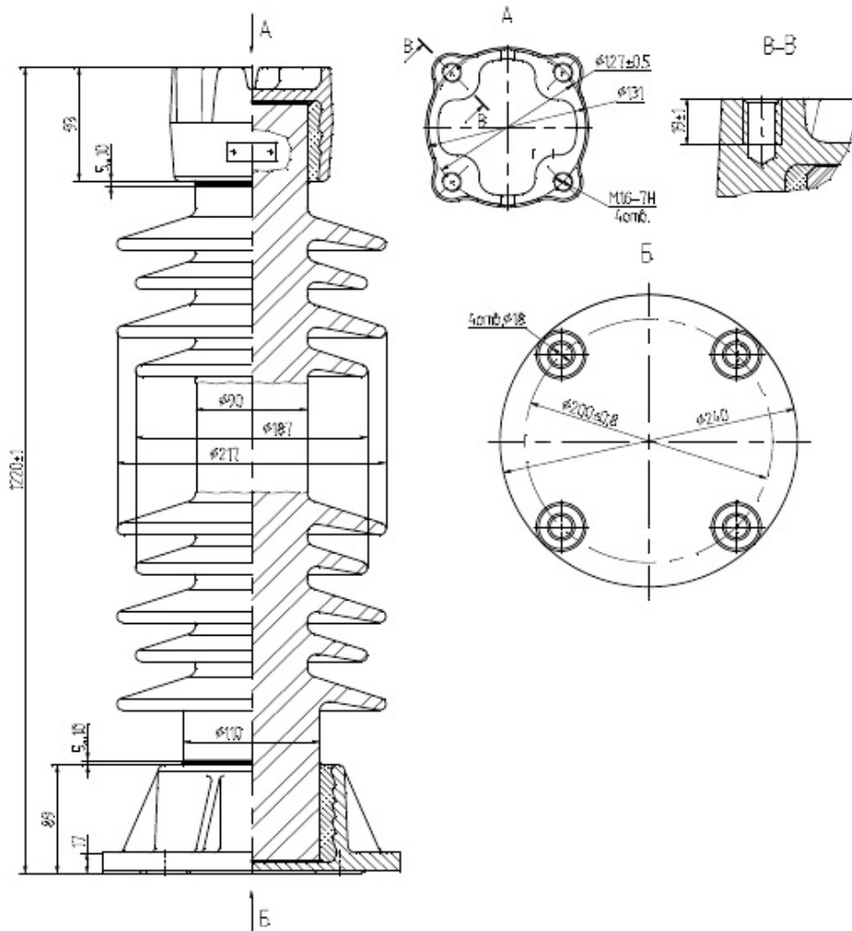
С4-550 II-М УХЛ 1 чертёж НИЮД.686144.011 СБ креслення
