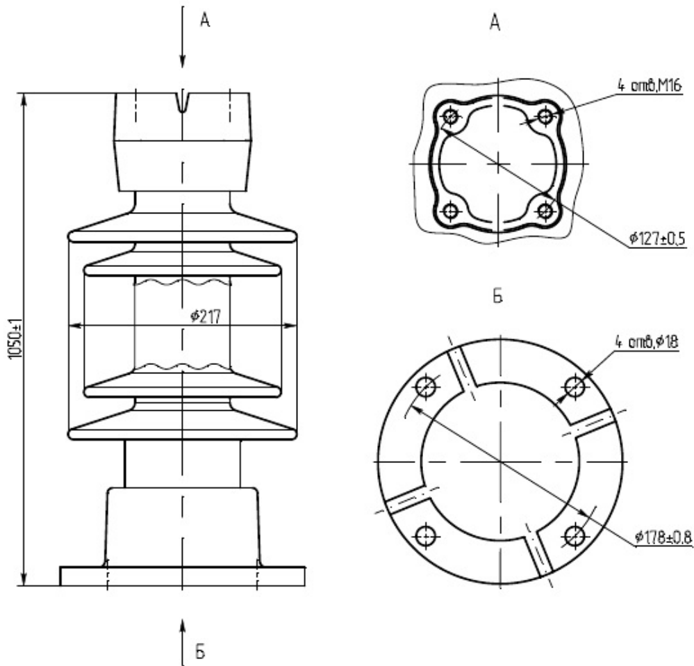
С4-450 II-M УХЛ1 чертёж НИЮД.686144.023 СБ креслення
